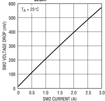
SW2 V_{\text{CESAT}}
